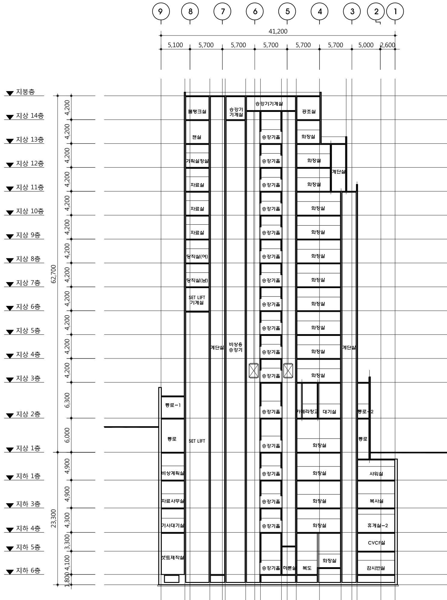
1 주 단 면 도 축척 : 1/400
