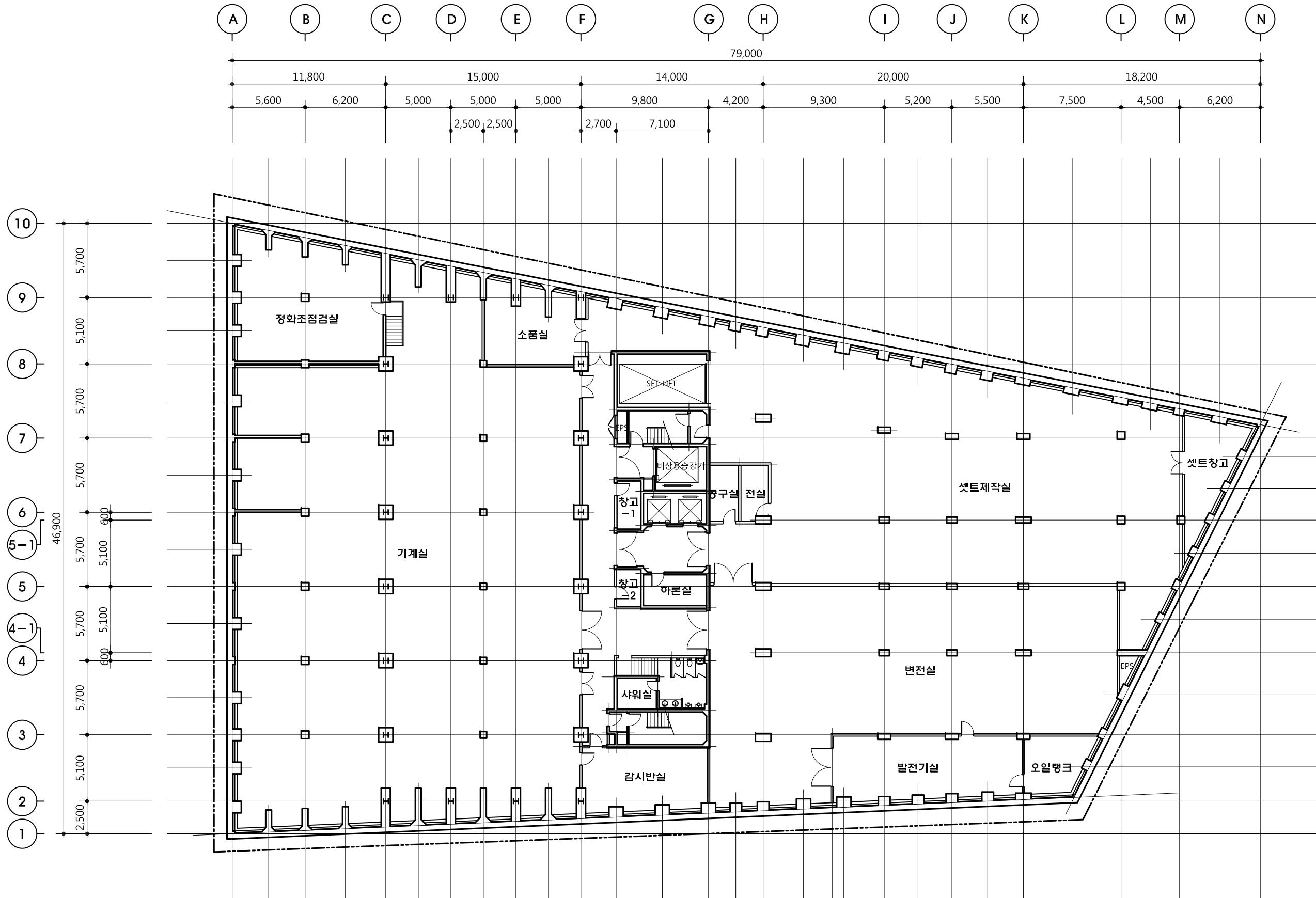
1 지하6층 평면도 축척 : 1/300
