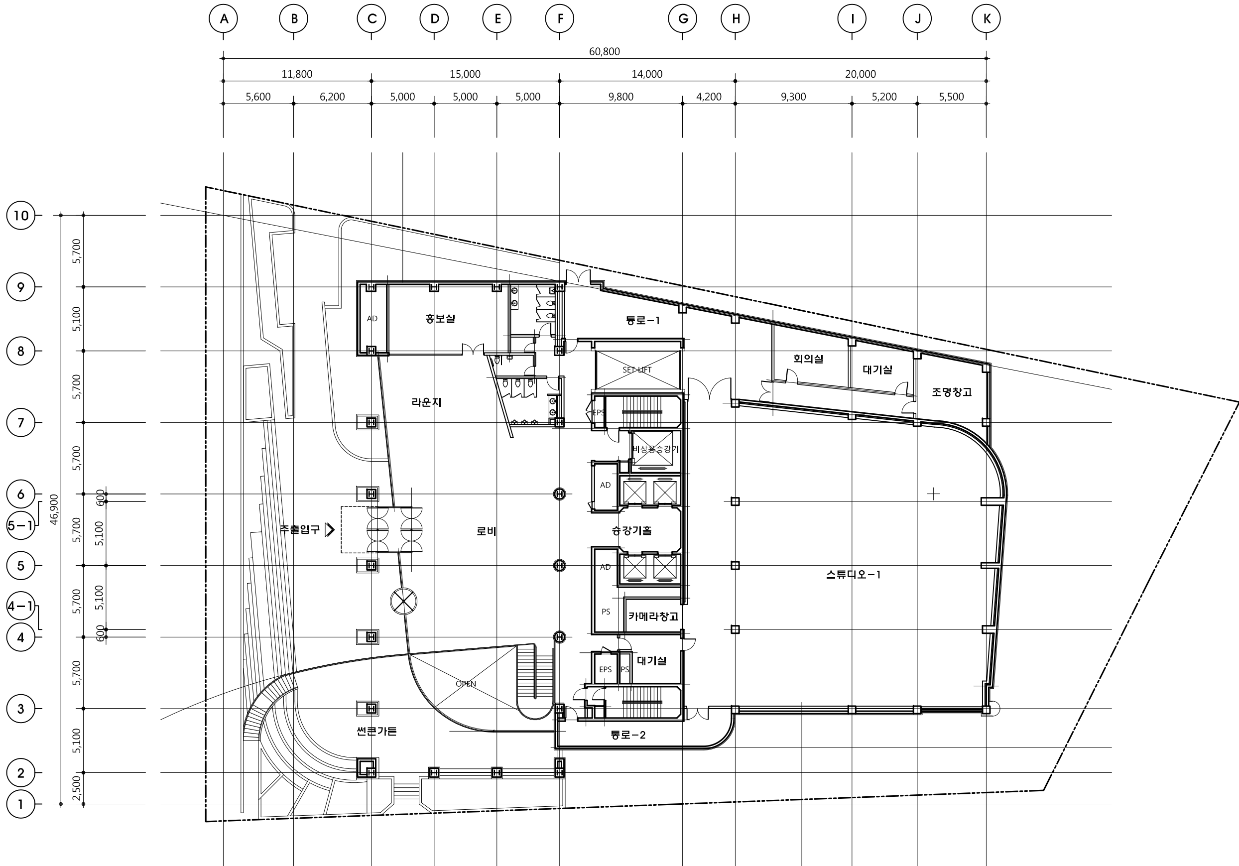
1 지상2층 평면도 축척 : 1/300
